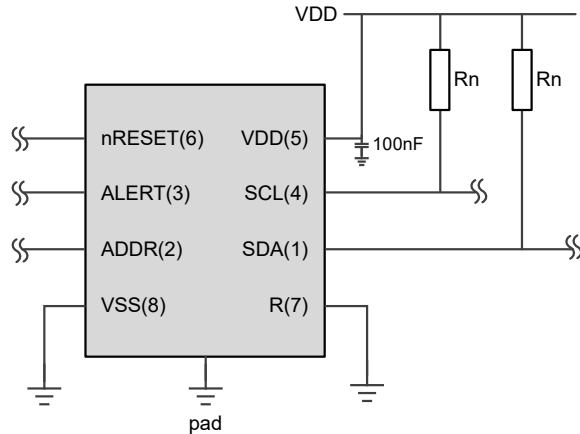
图 3 典型应用图
