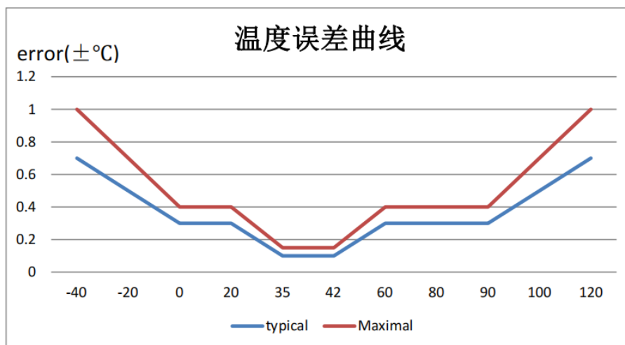
图 2 GXTS03 温度误差图
