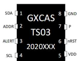
图 1 GXTS03 芯片效果图
