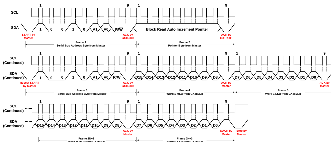
图 6 I 2 C 寄存器块读取时序图
