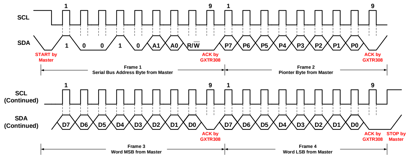
图 3 I 2 C 写命令时序图
