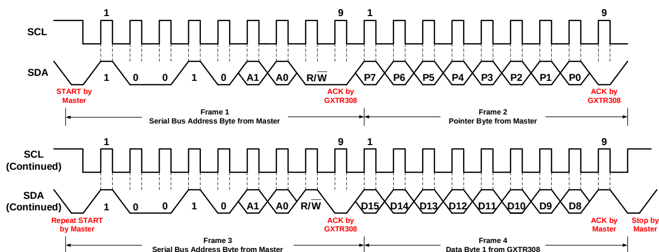
图 5 I 2 C 读命令（1 Byte）时序图
