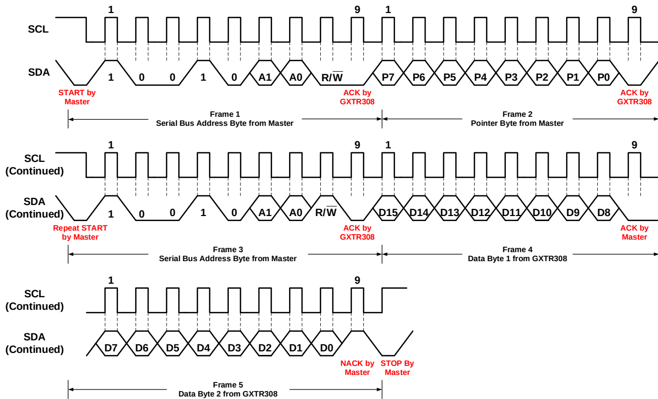
图 4 I 2 C 读命令 (2 Byte) 时序图
