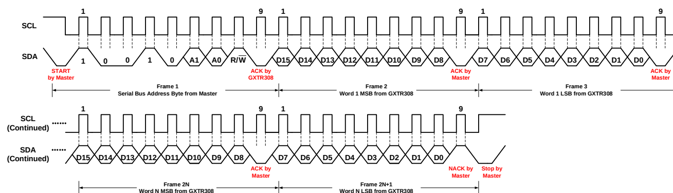
图 7 I 2 C 无需指针字节的寄存器块读取时序图
