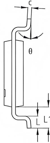
侧视图
