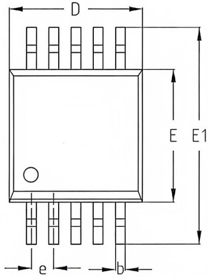
正视图
