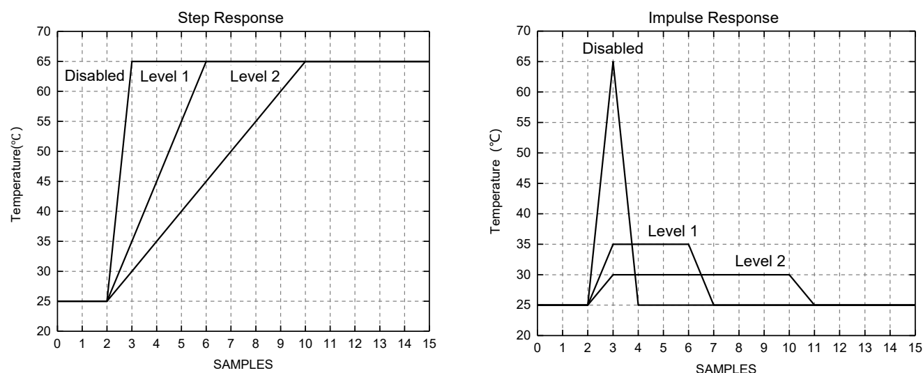
图 3 GXTR3032 中可编程数字滤波器工作示意图
