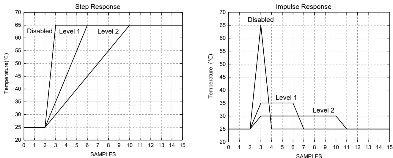
图 3 GXTR3012 中可编程数字滤波器工作示意图
