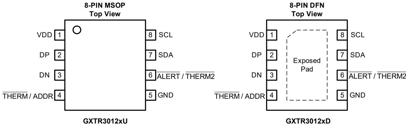
引脚功能
