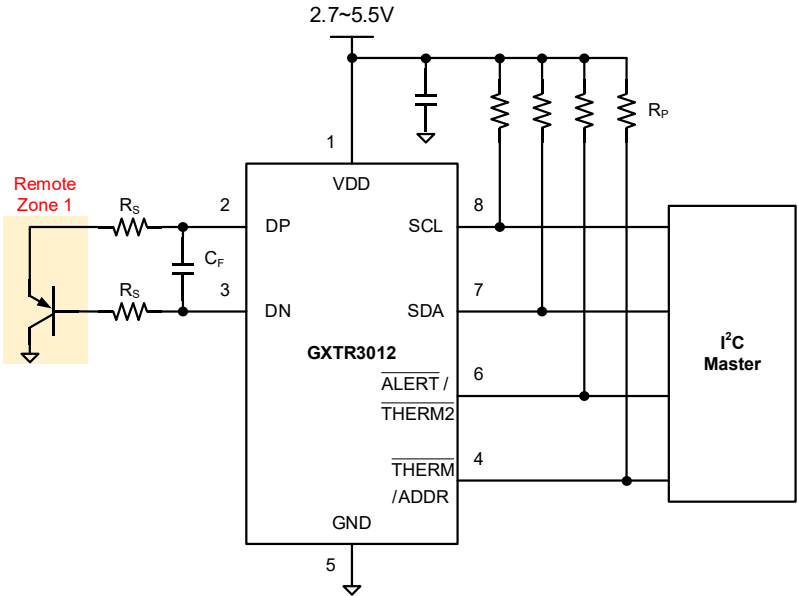
图 1 GXTR3012 典型连接示意图
