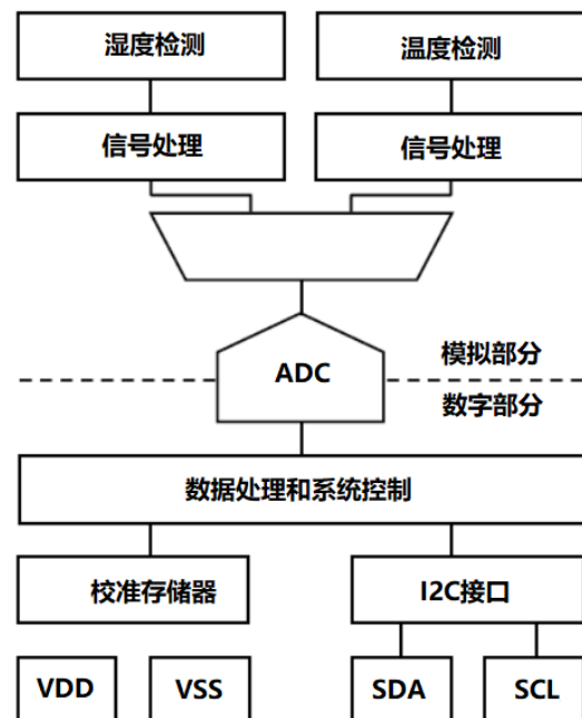
图 2 GXHTV3 功能原理框图
