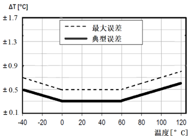
图 5 GXHTV3 温度误差图
