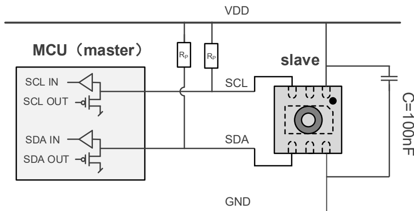
图 7 GXHTV3 的典型应用电路 (包括上拉电阻和去耦电容)。
