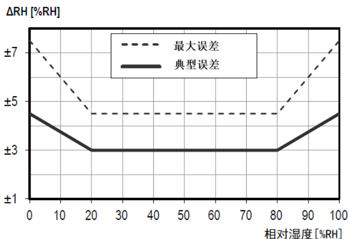
图 3 GXHTV3 湿度误差@25°C
