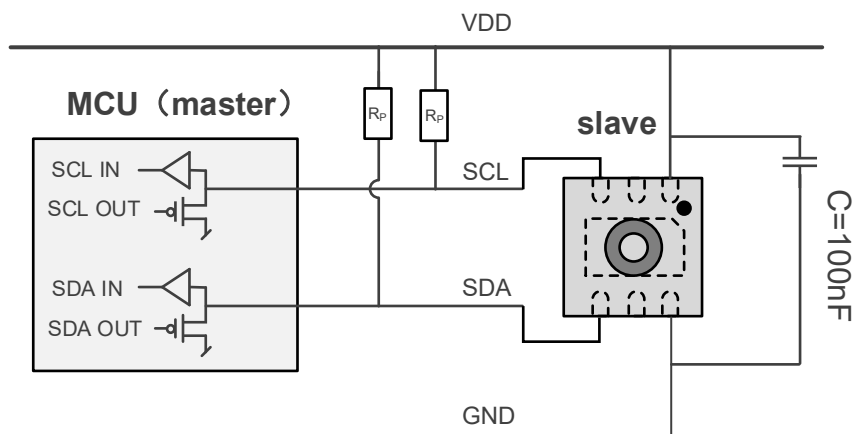
图 7 GXHTC3 的典型应用电路 (包括上拉电阻和去耦电容)。
