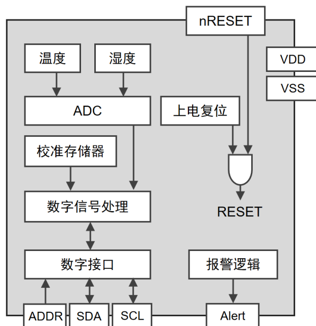
图 2 GXHT31 功能原理框图
