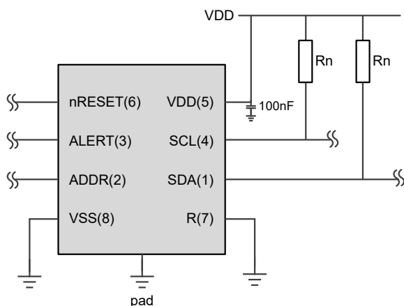
图 6 典型应用图
