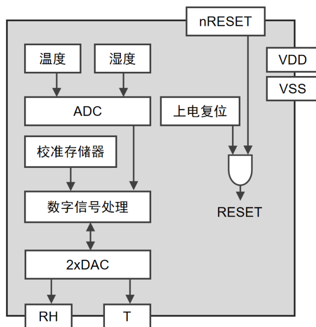
图2 GXHT30A 功能原理框图
