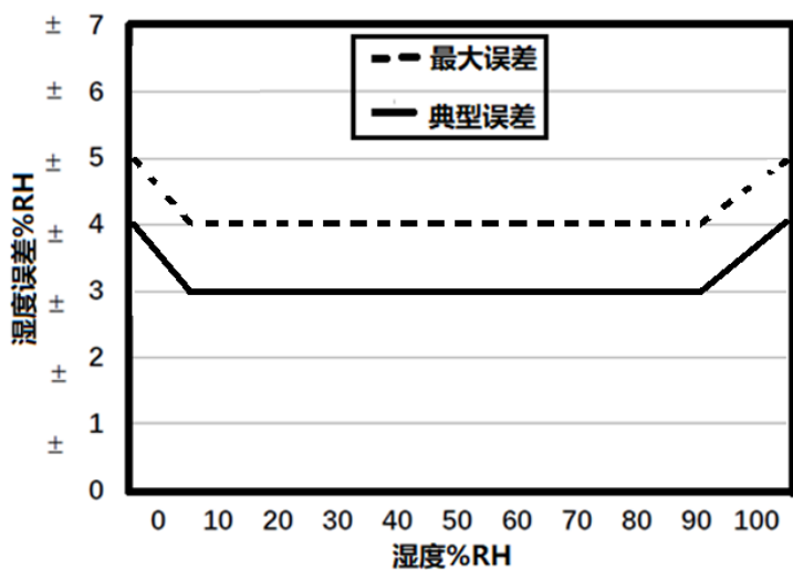
图 3 GXHT30 湿度误差@25°C
