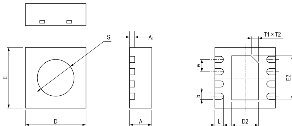
图 7 GXHT30 传感器封装尺寸
