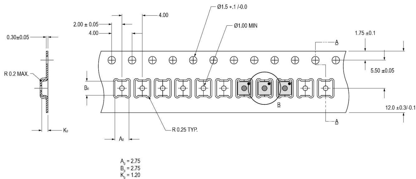
图9 芯片运输用编带尺寸说明
