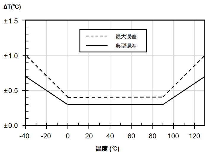
图 4 GXHT30 温度误差图
