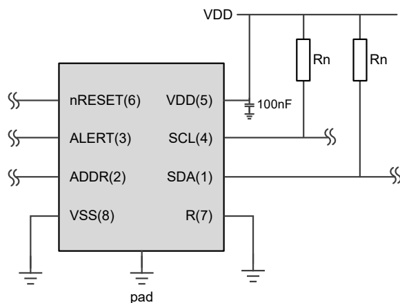
图 5 典型应用图
