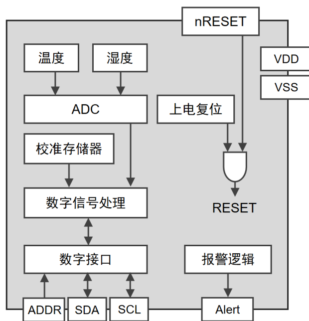
图 2 GXHT30 功能原理框图
