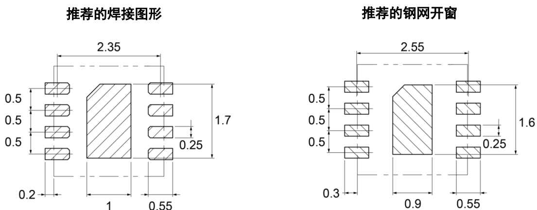
图 8 推荐的焊接图形和钢网开窗图形（灰色虚线代表 DFN 的封装外形）
