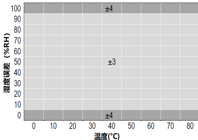
图 3.1 不同温度条件下 GXHT30 的误差
