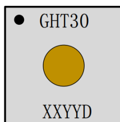
图 6 GXHT30 顶视图及激光标记
