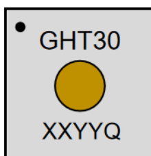
图 6 GXHT30 顶视图及激光标记
