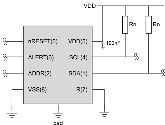
图 5 典型应用图
