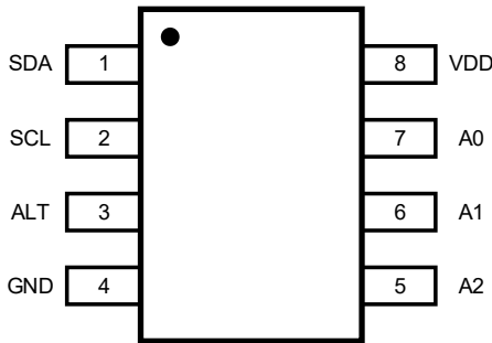
引脚功能
