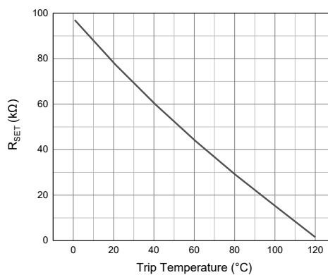
R_{set} 与触发温度的关系
