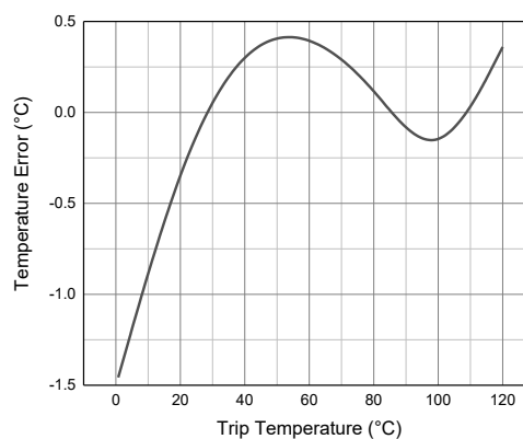
温度误差与触发温度的关系
