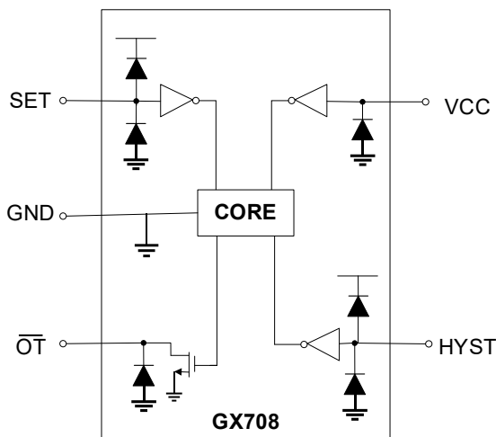
GX708 内部 ESD 等效电路
