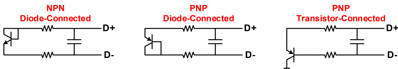
图 8 GX451 远程测温探头连接方式
