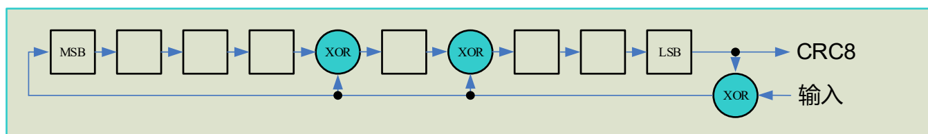
图 9. CRC 产生器
