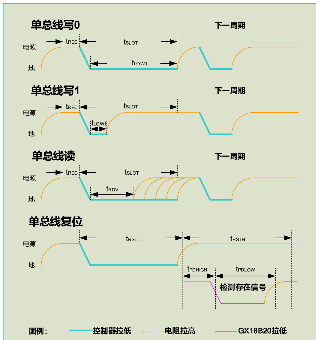
图 18. 时序
