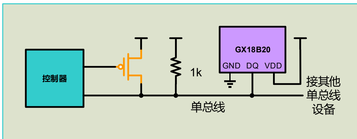
图 5. 使用外部电源为 GX18B20 供电
