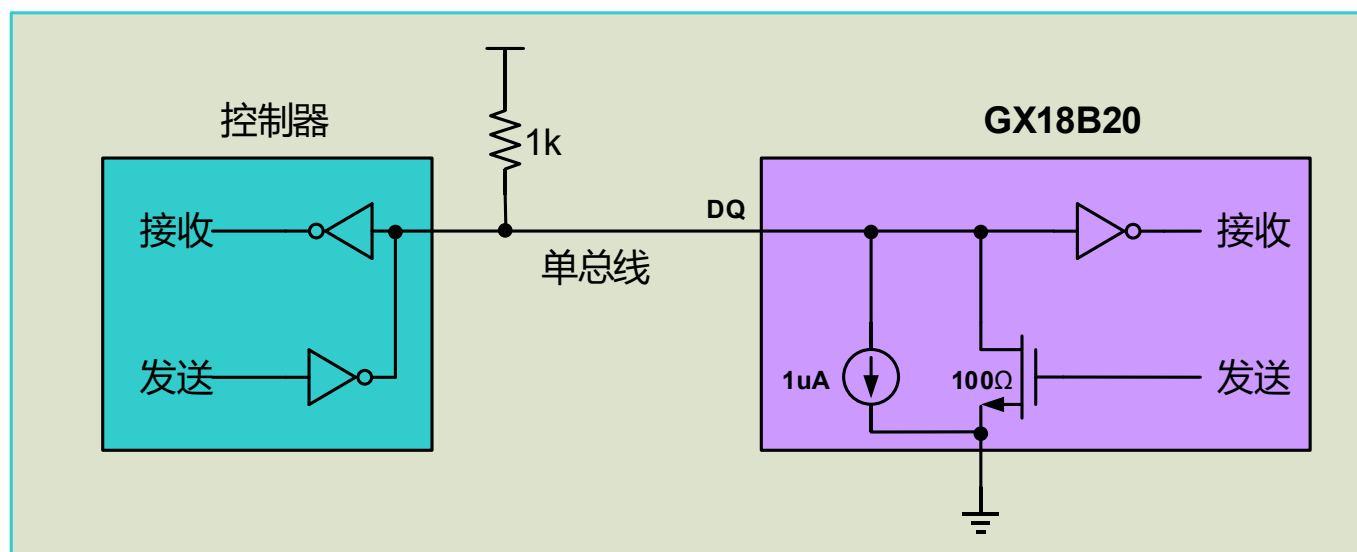
图 10. 硬件结构图
