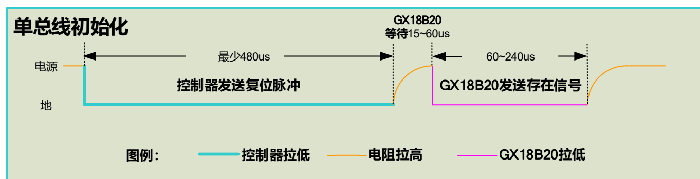
图 13. 初始化序列
