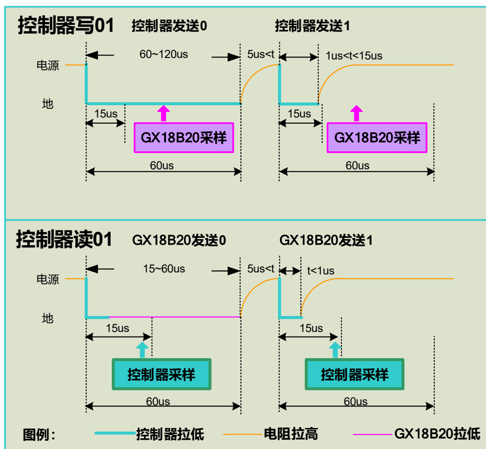
图 14. 读/写时序图
