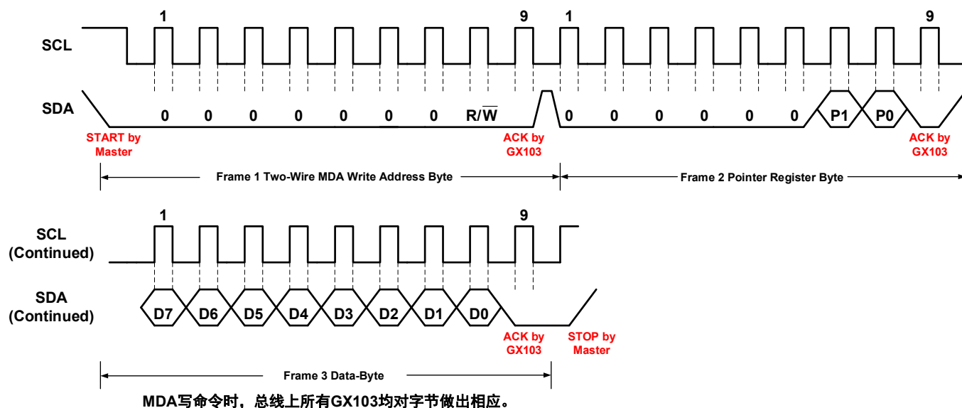
图 6 两线制 MDA 写命令时序图
